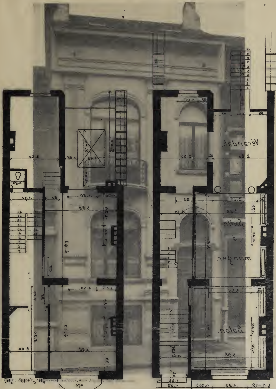
Maison de M. X., rue de Rotterdam, 5
